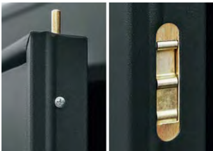
Feststellmechanik der 2-flügeligen Türen
