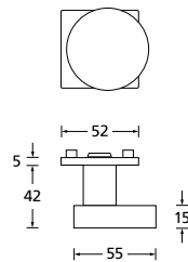
Knopf zyl. versetzt
