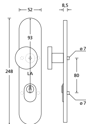
Zylinderüberstand: 11-16 mm
