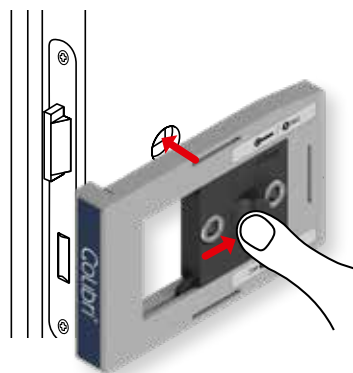
Bohrschablone für Schlüsselrosetten
