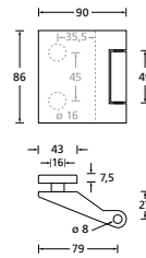
Glastürband Paar Glastürband 3-teilig
